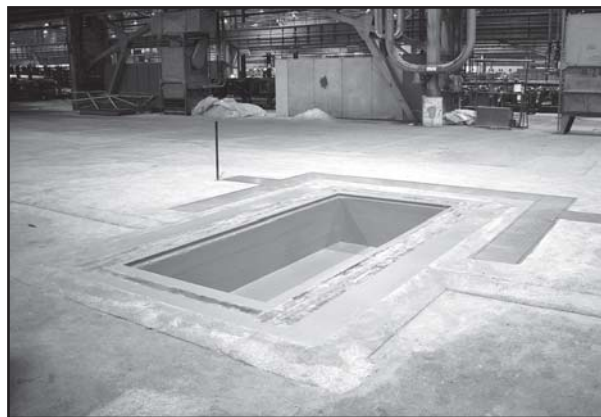
Základ desaťvalcovovej rovňacky - pripravovanej finalizáčnej linky výmenníkových rúr. F: A.Nociarová
